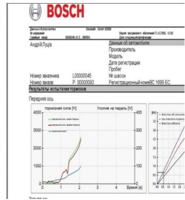
Рис. 1. Загальний вигляд роликів гальмівного стенда BSA 4340 (а) та можливий вивід результатів діагностування гальм автомобіля
