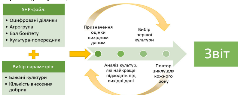
Рисунок. Схема послідовності роботи алгоритму
