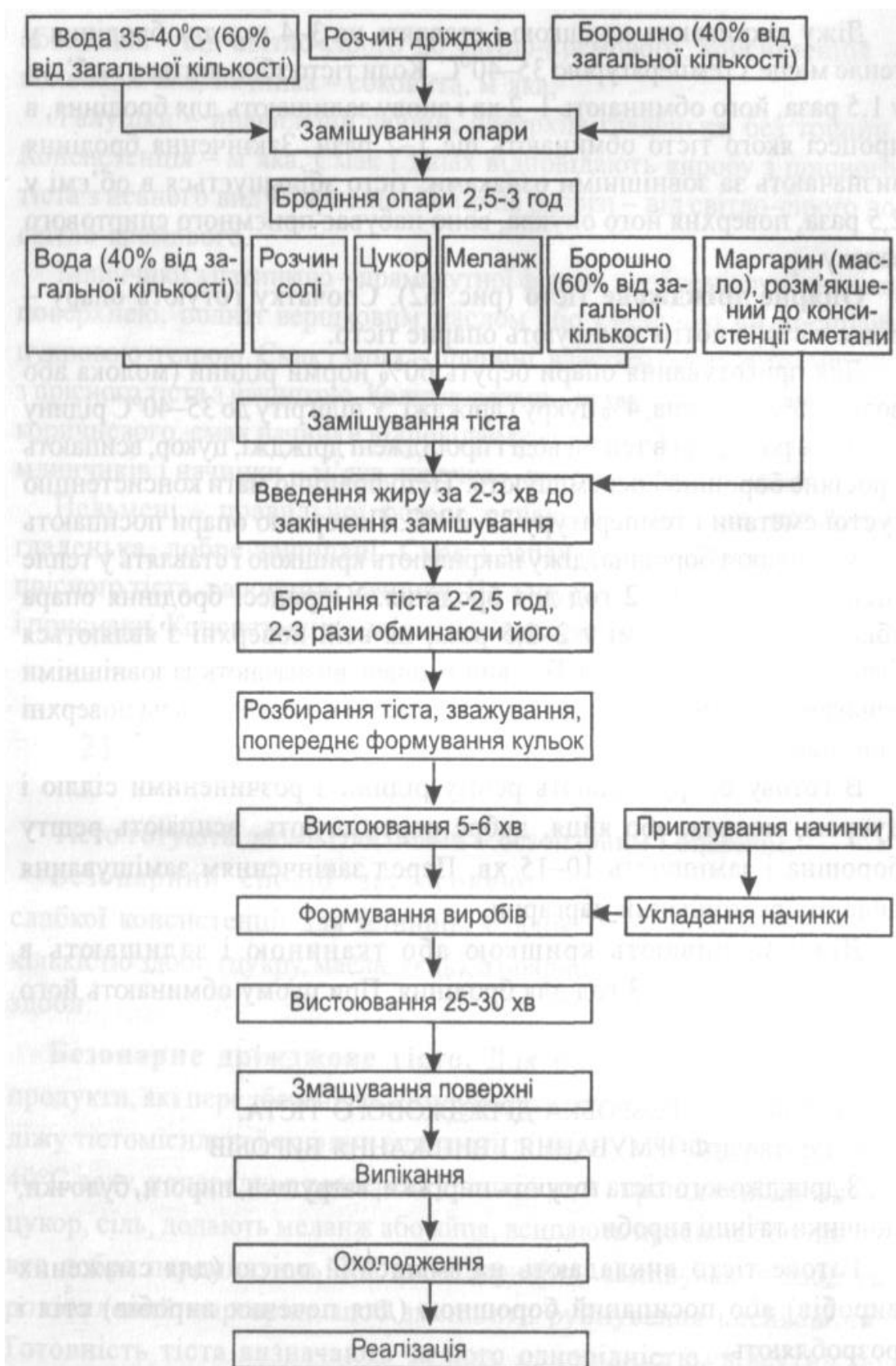
Рис. 1. Технологічна схема приготування виробів з дріжджового тіста (опарний спосіб)
