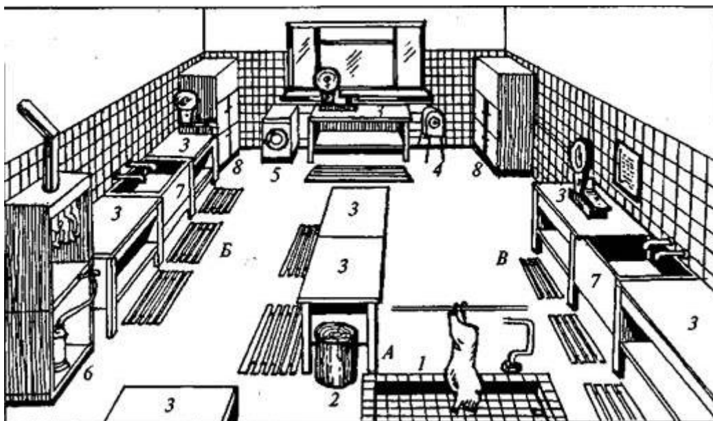
Рис 1 Розміщення обладнання у м'ясо-рибному цеху: А – дільниця обробки м'яса, Б – дільниця обробки птиці, В – дільниця обробки риби: 1 – ванна з бортиками, 2 – розрубувальна колода, 3 – столи виробничі, 4 – універсальний привід ПМ-1, 5 – м'ясорубка, 6 – обсмалювальна шафа, 7 – ванни мийні, 8 – холодильні шафи
