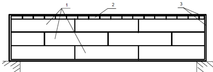
Рис.1. Схема комбинированной перемычки из легкогобетонных блоков (с перевязкой швов) и кирпича глиняного. 1 – газобетонные блоки; 2 – кирпич глиняный; 3 – обойма из углеродной ленты
