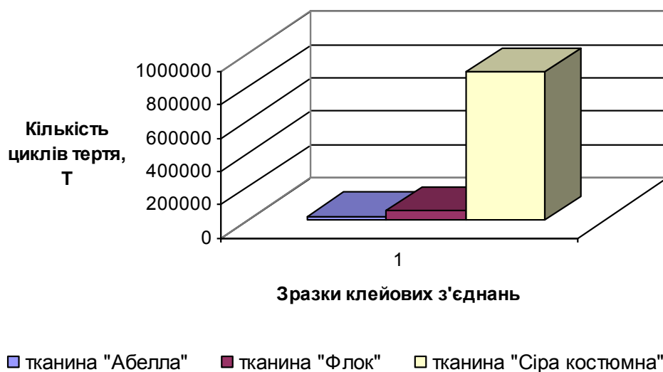
Рис.1. Діаграма оцінки тертя клейових з'єднань (клей UM-32)
