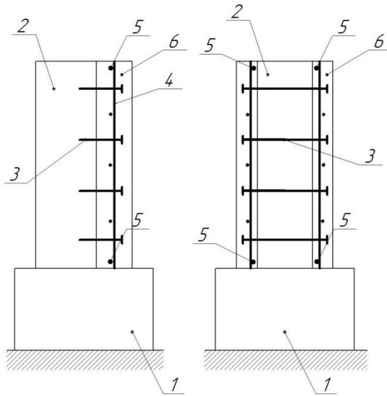
Рис. 2. Схема пристрою односторонньої (а) і двосторонньої (б) залізобетонних плит
