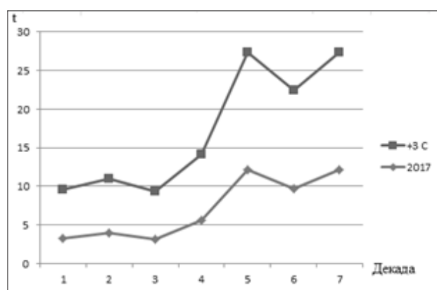
Рис. 1. Динаміка середньої за декаду ефективною температури
