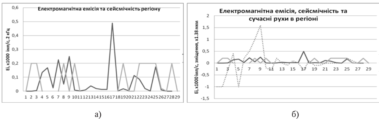
Рис. 1.2.: а) електромагнітна емісія в діапазоні 2 кГц (крива чорного кольору), сейсмічність (діаграма сірого кольору) Закарпатського внутрішнього прогину в лютому 2017 року; б) електромагнітна емісія (крива чорного кольору), сейсмічність (крива сірого кольору), сучасні горизонтальні рухи кори (пунктирна крива). Лютий 2017 року. РГС «Тросник», ПДС «Королево»
