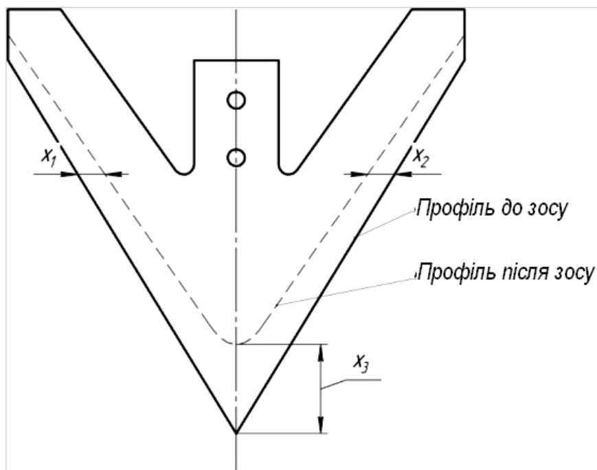
Рисунок 1. Схема вимірювання зносу лапи.
